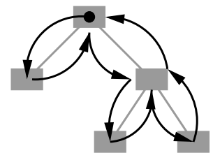
An Euler tour.
