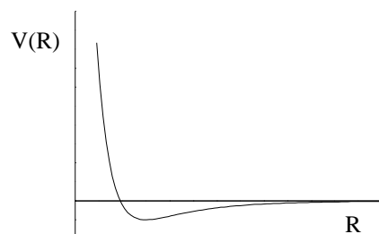
He - Lennard Jones \Delta \ll kT (T ambiente)
