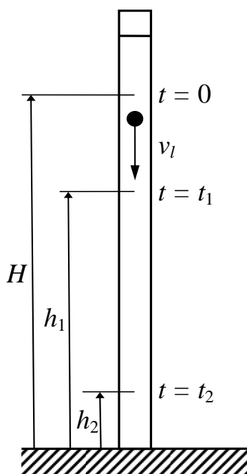
Figura 2: Esquema del dispositivo experimental
