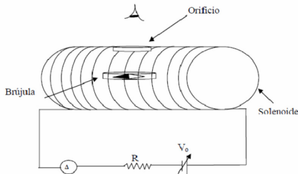
Figura 2: Esquema del dispositivo experimental
