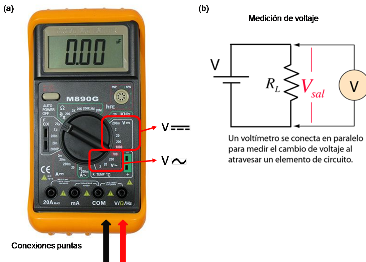
Figura 2: configuración para función de medición de voltaje.
