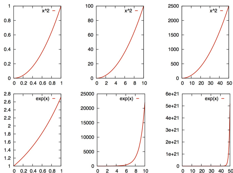
Figura 1: Comparación entre funciones potenciales (por ej. x^2 ) y no potenciales (por ej. \exp(x) )
