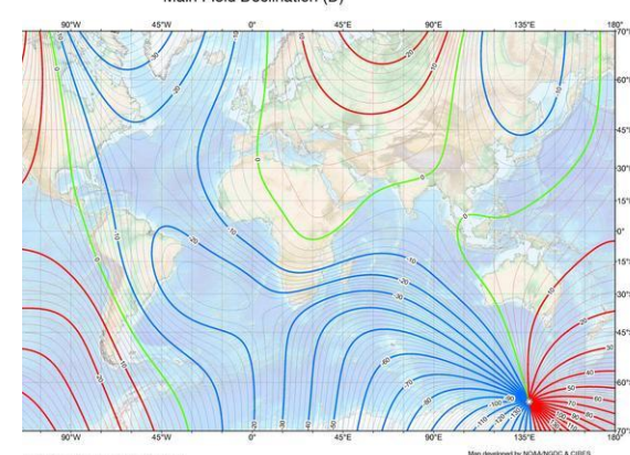
US/UK World Magnetic Model -- Epoch 2010.0 Main Field Declination (D)
