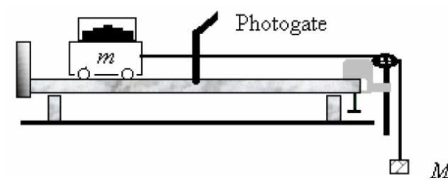
Figura 2 Esquema experimental propuesto.
