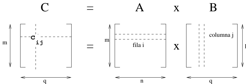
Figura 2.1: Multiplicación de matrices.
