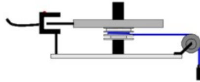
Fig.2: Montaje a emplear para el estudio del disco en rotación con torque externo
