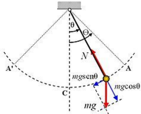
Figura 1: Diagrama de cuerpo libre del péndulo simple ideal. Atributo de imagen:
