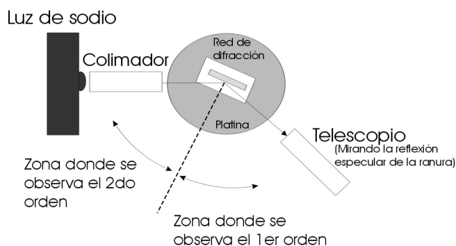
Figura 1. Esquema del dispositivo. Note la ubicación de la red respecto del haz proveniente de la lámpara de Na.
