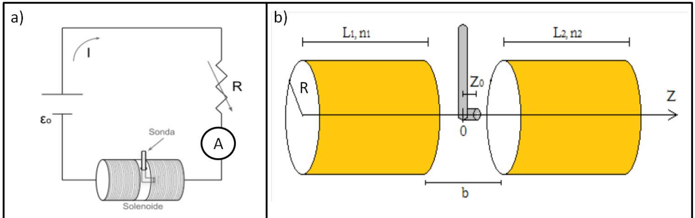
Figura 2: a) Esquema del circuito. b) Detalle de la bobina y la sonda hall, donde L_1=L_2=(11.3\pm 0.1) cm, R=(4.9 \pm 0.1) cm, n_1=n_2=(1000\pm 1) espiras/m y b=(3.1\pm 0.1) cm
