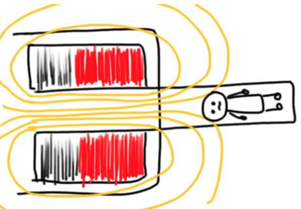
Aplicación de ondas de radiofrecuencia
