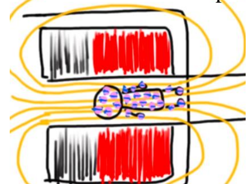
Alineación del spin de átomos de H con campo B
