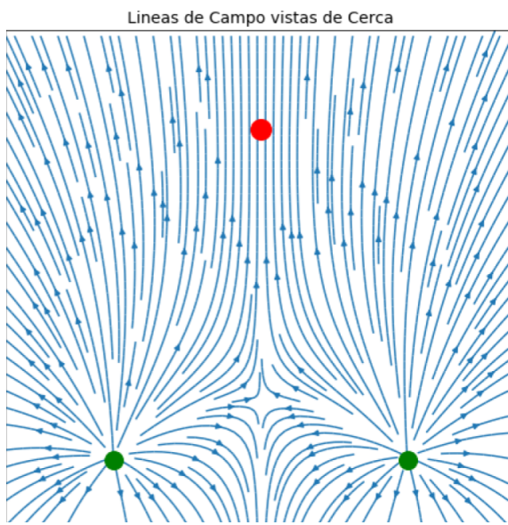
(c) Campo de cerca reemplazando la carga -3q por -2q
