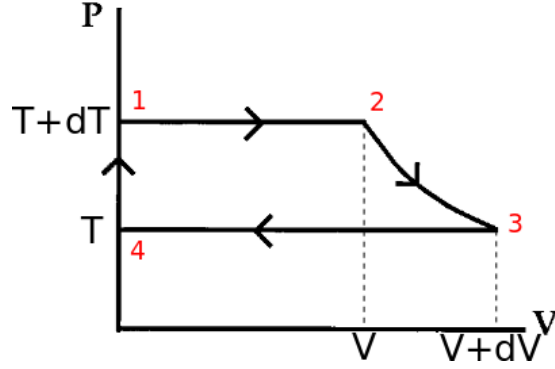
Figure 2: Diagrama P-V del ciclo de Carnot para el gas de fotones. Notemos que las isotermas son también isobaras, que la expansión isotérmica se da desde un volumen nulo, y que la adiabática se da solo en dV .
