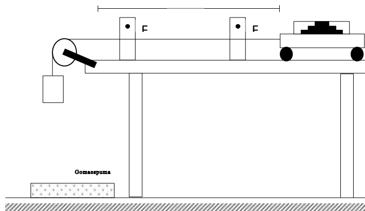
Figura 1: Esquema del montaje del experimento utilizando una polea, un hilo y una masa.
