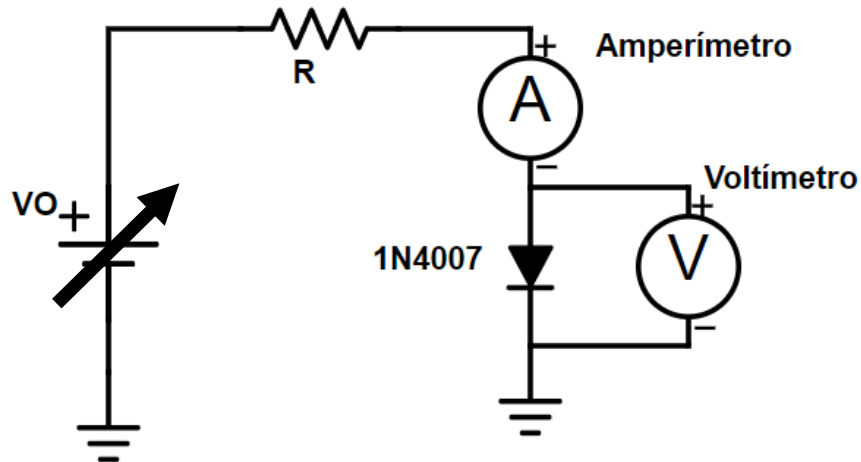
Medición con el diodo en directa
