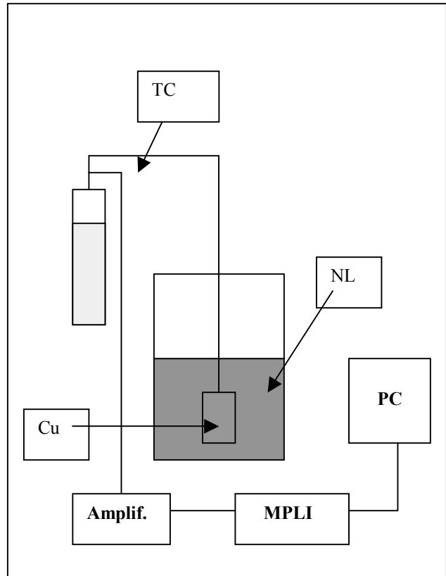
Fig.2. Arreglo experimental.
