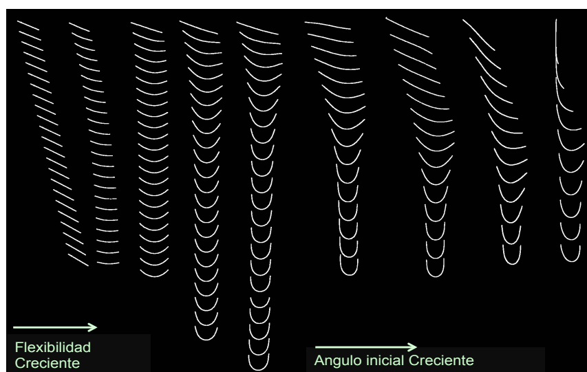
Cronofotografías de la sedimentación de una fibra flexible. Todos los filamentos tienen propiedades materiales similares (radio, densidad y módulo elástico).
