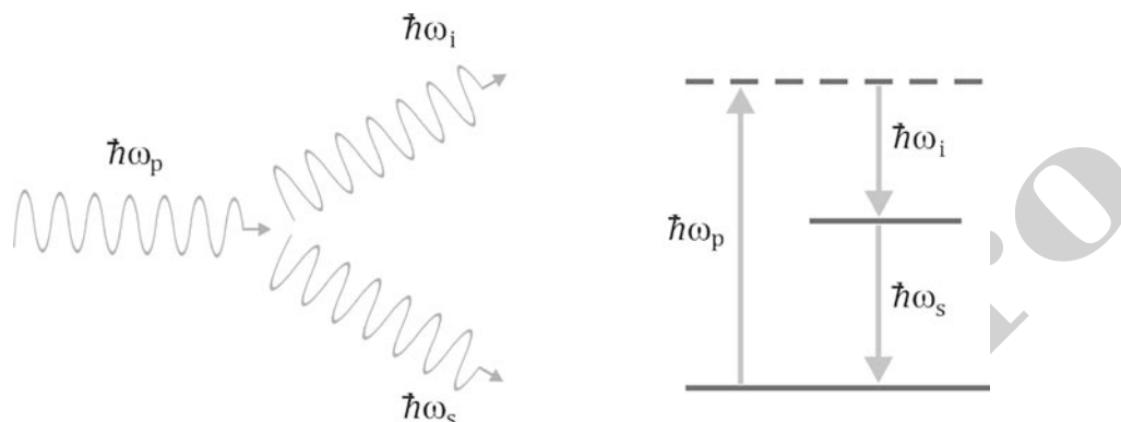
Figura1: Los esquemas representan la aniquilación de un fotón de alta frecuencia ( \omega_p ) y la creación de dos fotones de menor frecuencia ( \omega_i y \omega_s ) durante el proceso de fluorescencia paramétrica.
