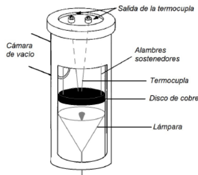
Figura 1: Esquema del dispositivo experimental
