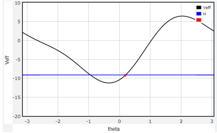
Figura 2: Forma funcional del potencial efectivo con gravedad. El equilibrio estable se desplaza hacia menores valores de \theta = 0
