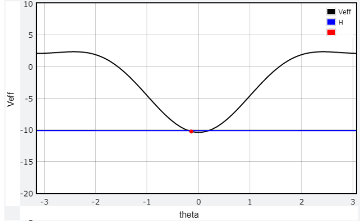
Figura 1: Forma funcional del potencial efectivo sin gravedad. El equilibrio estable es en \theta = 0 y \theta = \pi . En \theta = 2,41 hay un máximo.
