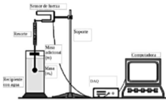
Figura 1: Esquema del dispositivo a utilizar en la práctica. El recipiente con agua se emplea sólo en la segunda parte .
