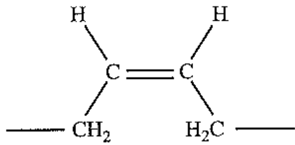
cis
