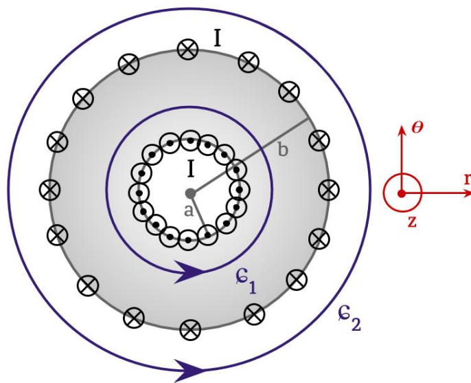
Figura 2: Toroide visto desde arriba con las curvas C_1 y C_2 de Ampere en distintas regiones del espacio
